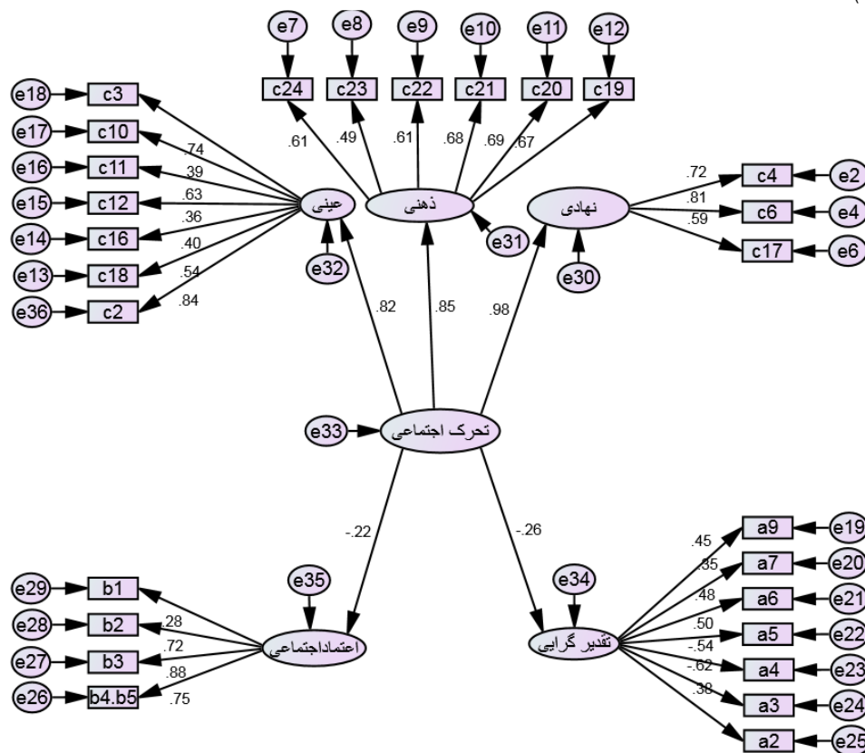
شکل ۲ - مدل مفهومی اولویت بندی عوامل مؤثر بر تحرك بين نسلی مهاجران افغانستانی در شهر کاشان
