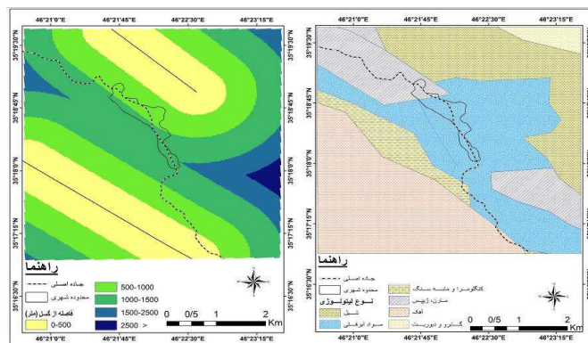
شکل ۵- پارامترهای زمین‌شناسی
